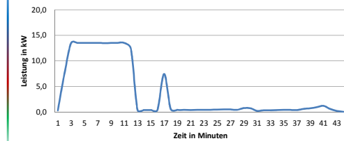
Leistungsabnahmeverlauf
