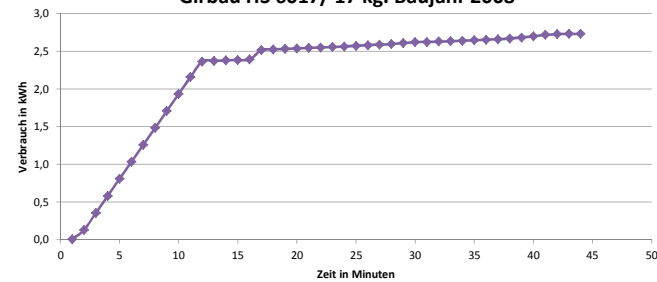
Energieverbrauchsmessung an der Waschschleudermaschine Girbau HS 6017/ 17 kg. Baujahr 2008
